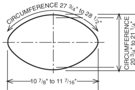
附图显示标准的球的长轴剖面。
